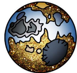
Pluto
